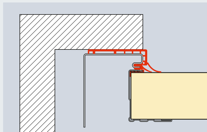
Mocowanie boczne z zastosowaniem ThermoFrame
