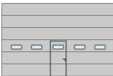
SPU F42 Okna segmentowe typ A Drzwi przejściowe usytuowane centralnie
