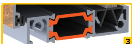
IZOLOWANY TERMICZNIE CIEPŁY PRÓG
