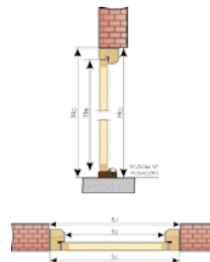
Linia Prima Thermo (ościeznica drewniana)
