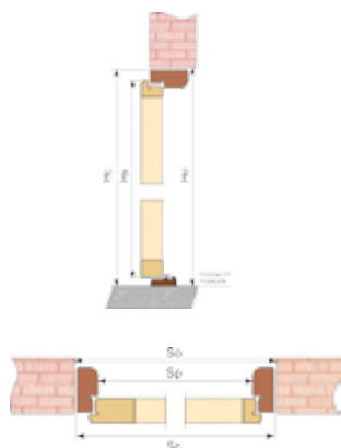
Linia Termika Felc (ościeznica drewniana)
