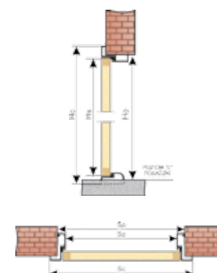
Linia Basic (ościeznica metalowa -połówkowa Basic)
