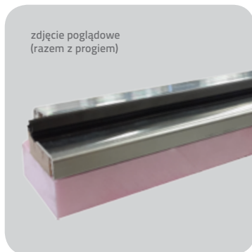
Poszerzenie podprogowe - wysokość 30 mm Poszerzenia można ze sobą łączyć na dowolną wysokość Cena: 39 zł netto
